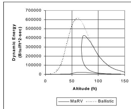
k. Dynamic Energy (Ftu/ft 2 -sec)
